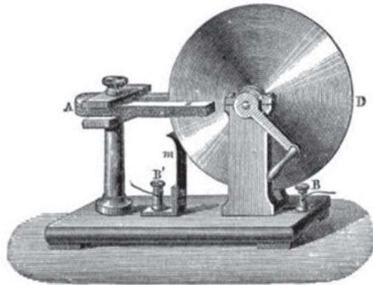
सन् १८३१ मा फाराडेले बनाएको पहिलो इलेक्ट्रिक जेनेरेटर
